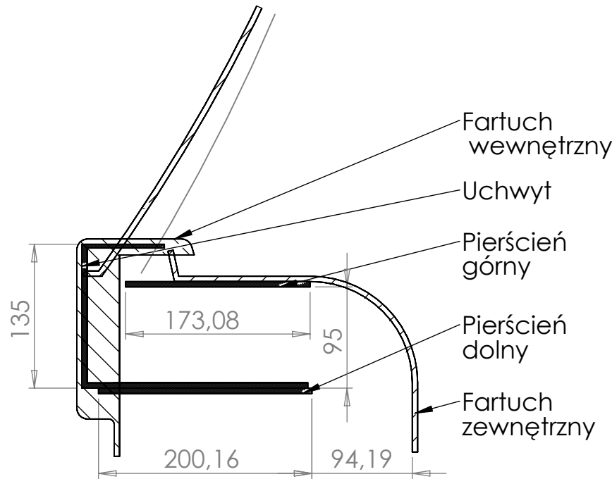
SZCZEGÓŁ A SKALA 1 : 5
